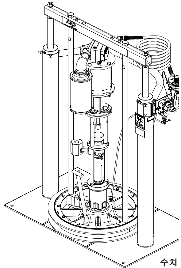
TP0665S5XXXXXXX 램 패키지
